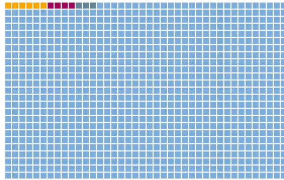
Klinische Testsensitivität = 60 %
